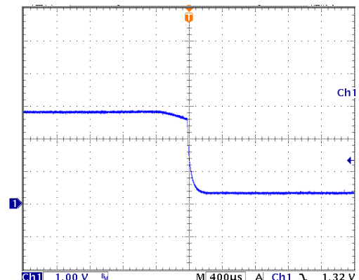
Vin=12V , Io=10A
